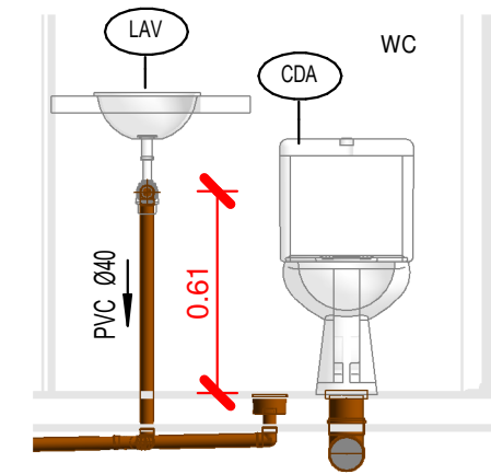
VISTA 03' - ESGOTO 1 : 25
