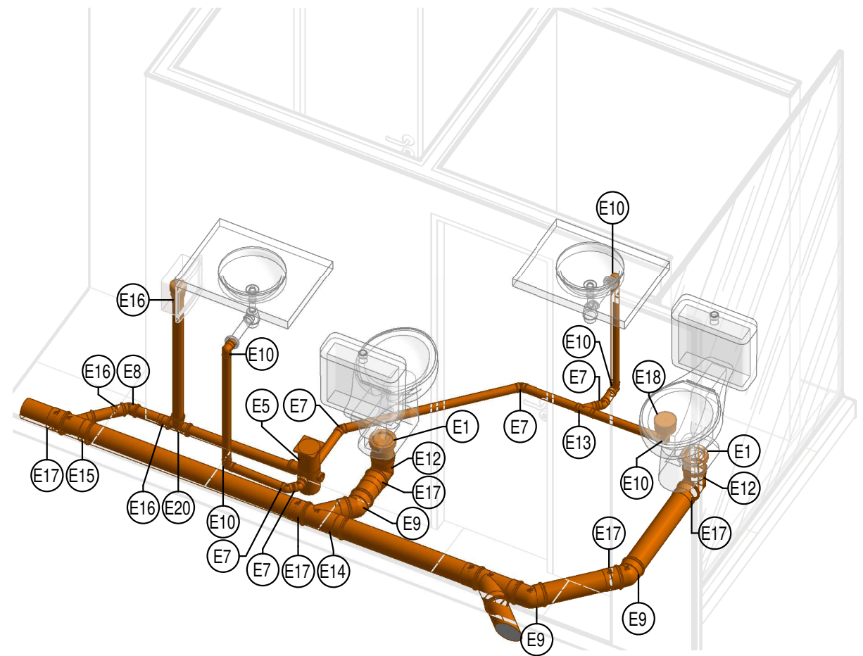
PERSPECTIVA 03 - ESGOTO
